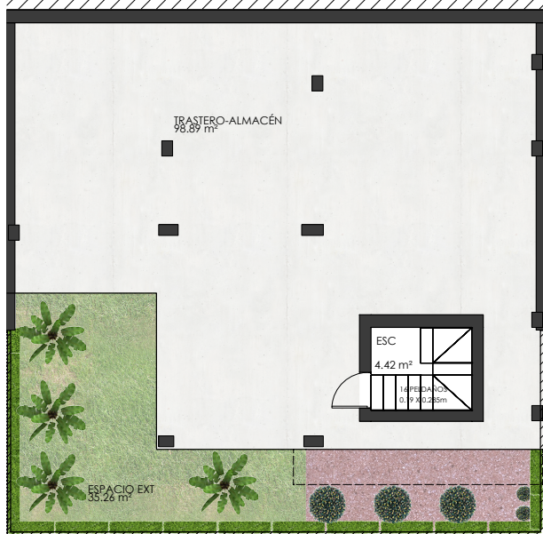
Planta Sótano
